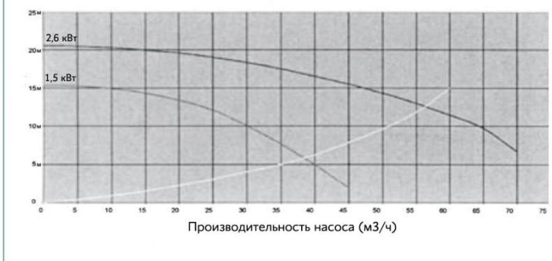
График работы насосов мощностью 1,5 кВт, 2,6 кВт
