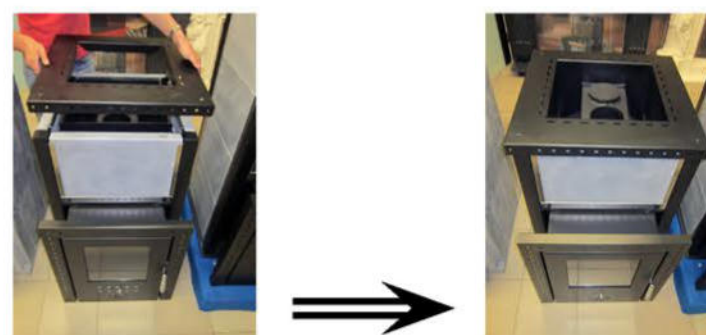
7) Установка верхней крышки.
